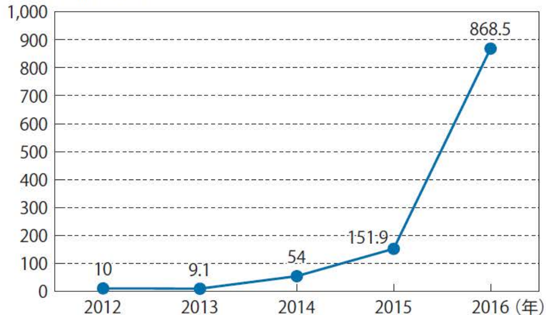
【宛先ポート「23/TCP」 (注)2 に対するアクセス件数の推移】
